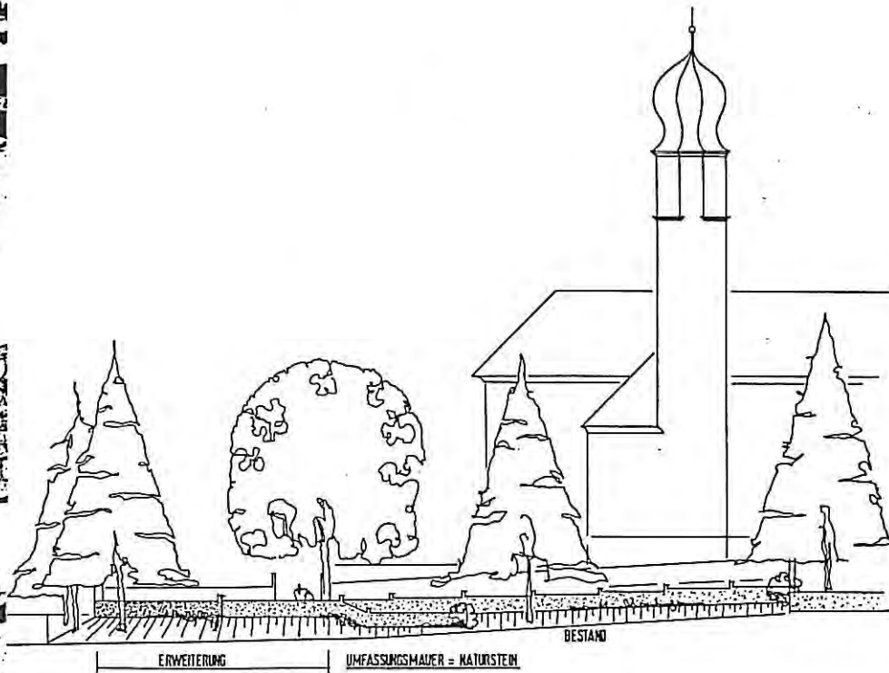
SÜDANSICHT
