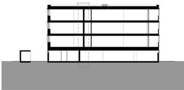
QUERSCHNITT (BAUTEIL A)
