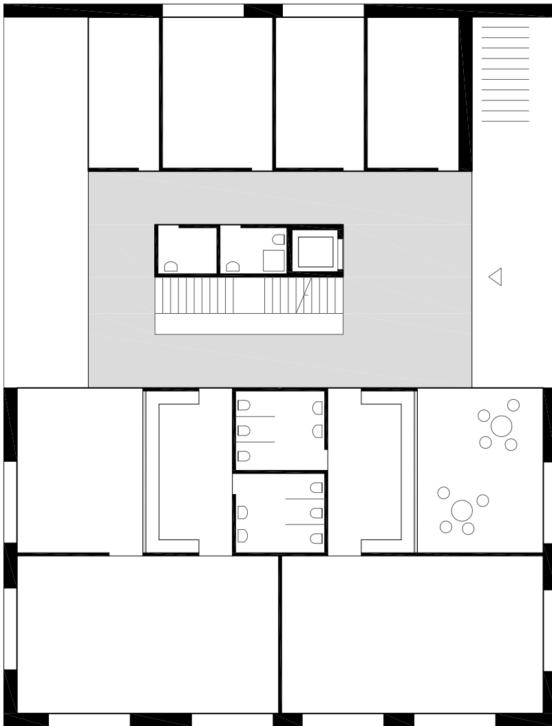
GRUNDRIB EG
