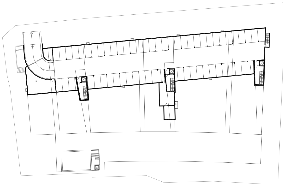
Grundriss Tiefgarage
