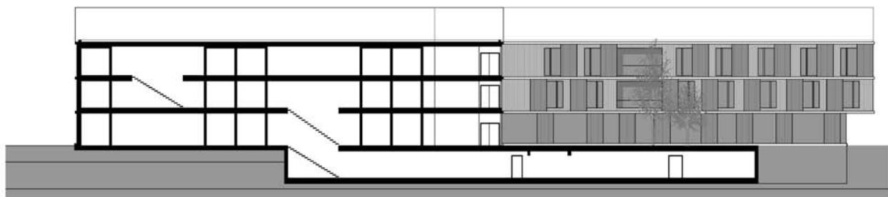
SCHNITT D-D
