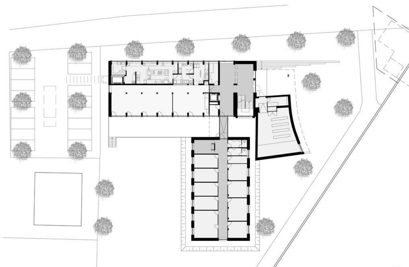
GRUNDRISS EG
