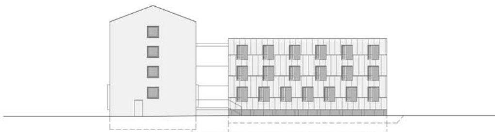
ANSICHT WEST
