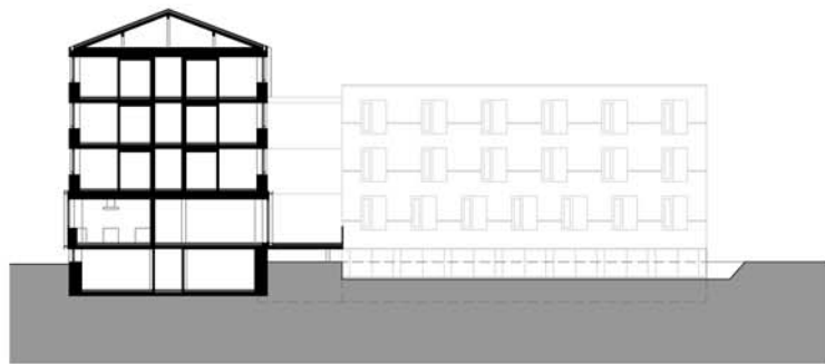
SCHNITT D-D
