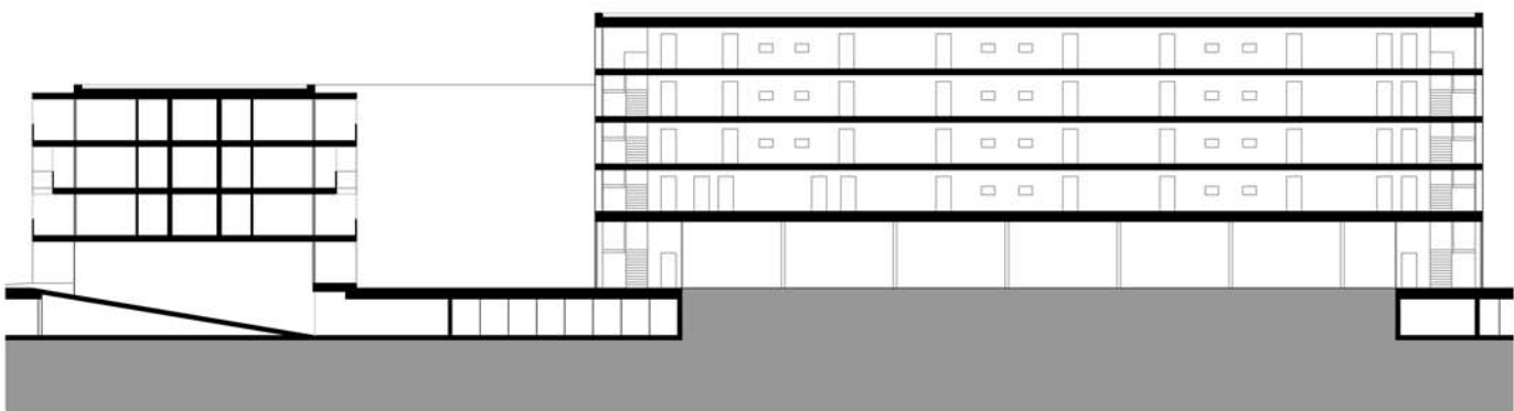
SCHNITT D-D
