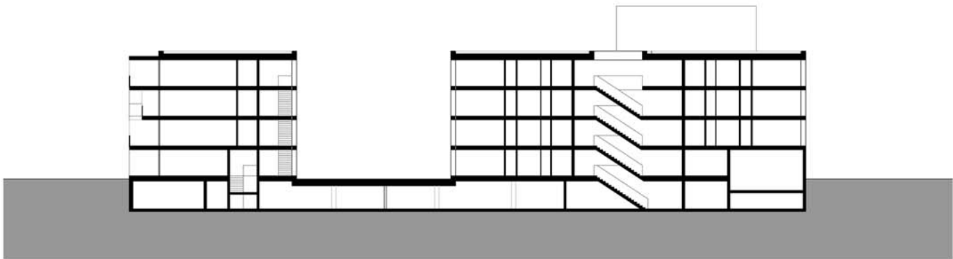
SCHNITT C-C
