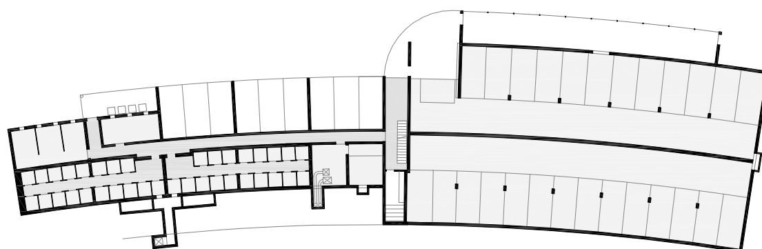
Untergeschoss
