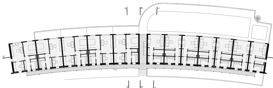
Erdgeschoss
