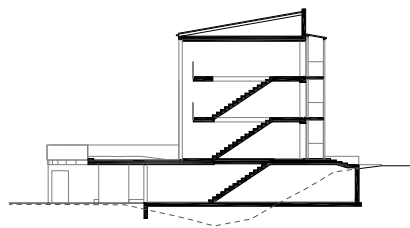
Schnitt B-B
