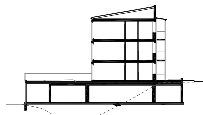
Schnitt C-C
