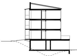
Schnitt A-A
