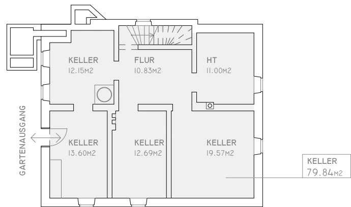
Kellergeschoß
