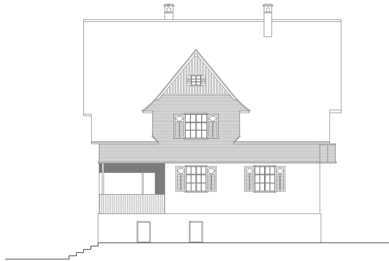
Ansicht Süd
