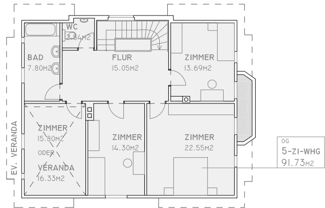
Obergeschoß
