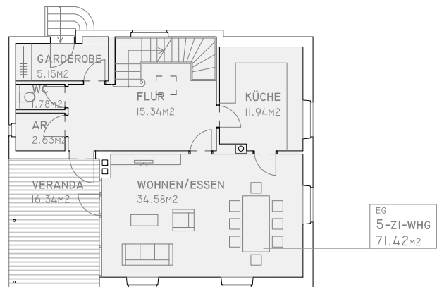
Erdgeschoß
