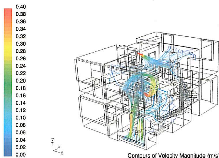
Abb. 5: Luftströmungen in m/s im zweigeschossigen Wohnraum des Passivhauses mit aktiviertem Parapet-Heizkörper. Grafik: arsenal research
