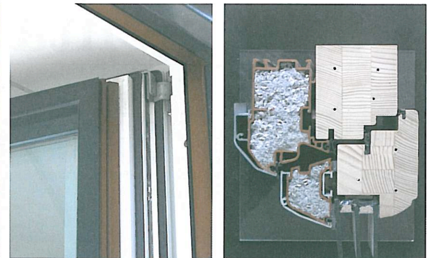
Abb. 14, 15: Geprüftes Passivhaus-Fensterprofil. Fotos: Hackermüller
